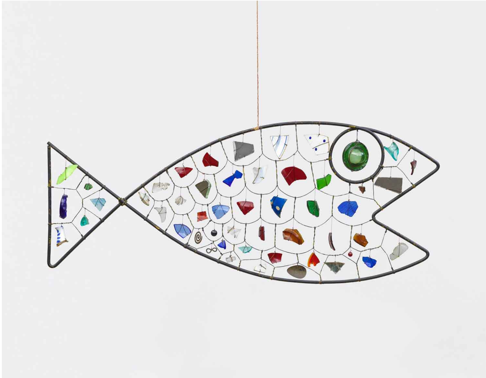
Poisson 1944
